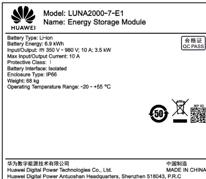
Rysunek 2-12 Tabliczka znamionowa modułu magazynu energii
