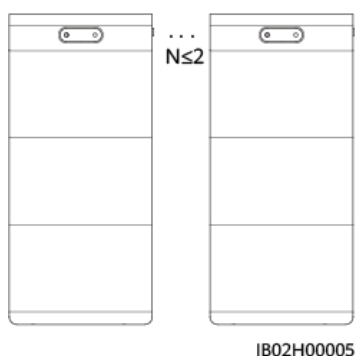
Rysunek 2-5 Połączenie równoległe
