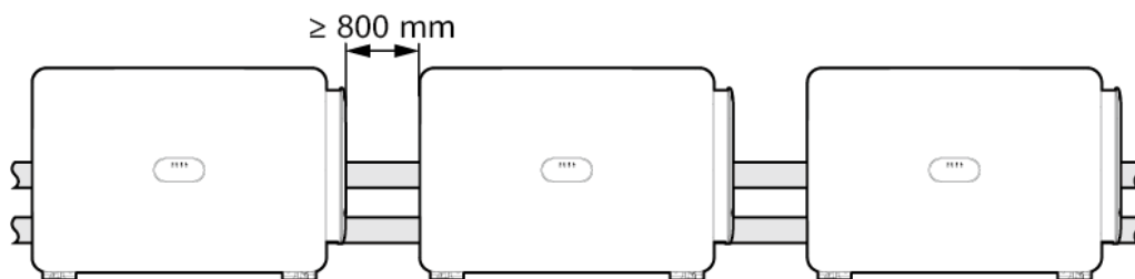
Rysunek 4-5 Montaż poziomy (zalecany)
