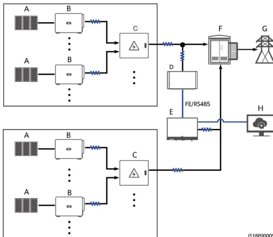
Rysunek 5-3 Zastosowanie sieciowe MBUS (transformator dwuuzwojieniowy + SmartMBUS CCO)
