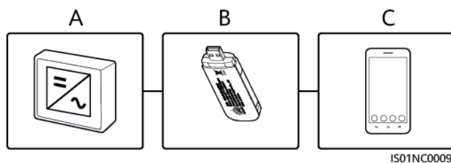
Rysunek 7-1 Podłączenie modułu WLAN
