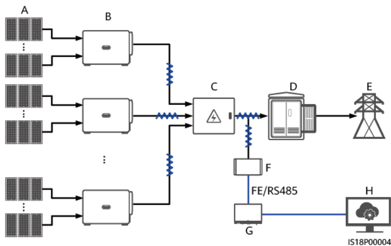
Rysunek 5-2 Zastosowanie sieciowe MBUS (transformator jednuzwojieniowy + SmartMBUS CCO)
