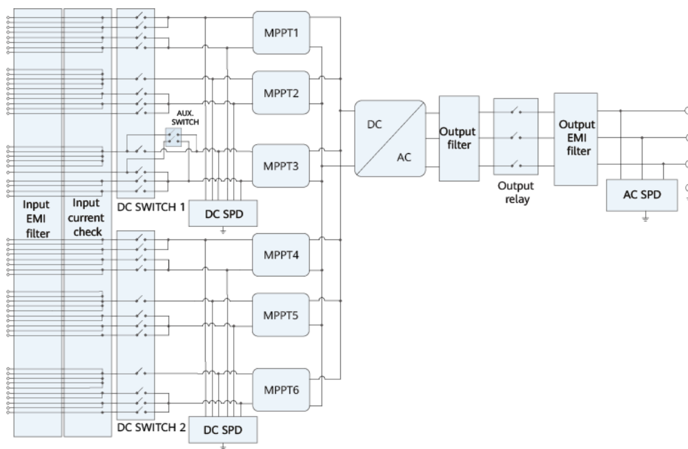
Rysunek 2-9 Schemat
