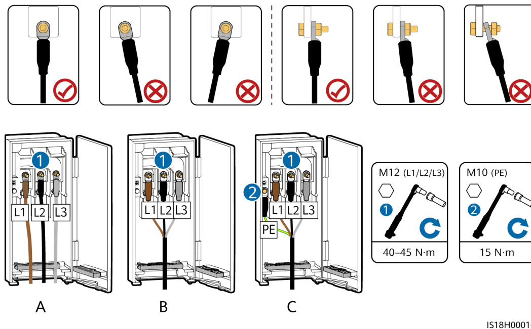
Rysunek 5-11 Podłączanie przewodu 1
