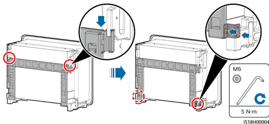
Rysunek 4-14 Zabezpieczanie SUN2000
